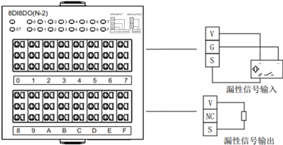
8DI8DO(N-2)
