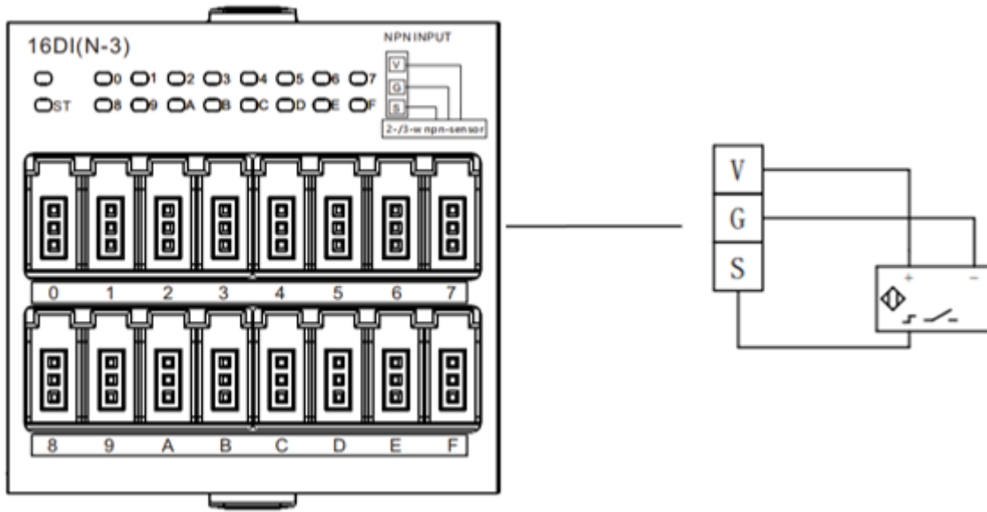
16DI(N-3)
