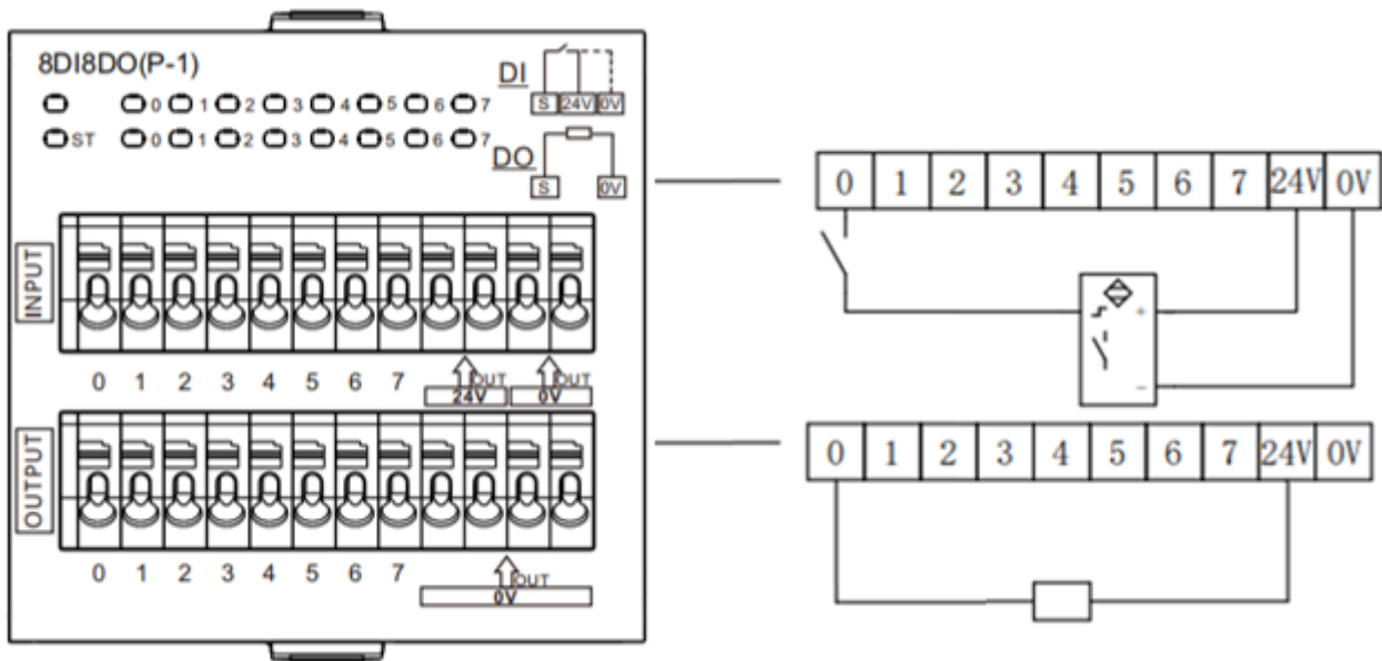
8DI8DO(P-1)
