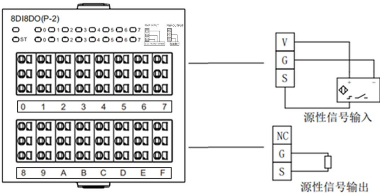
8DI8DO(P-2)
