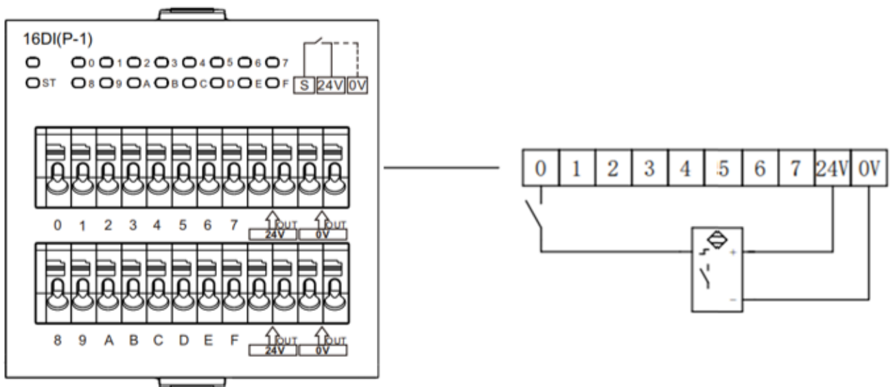
16DI(P-1)
