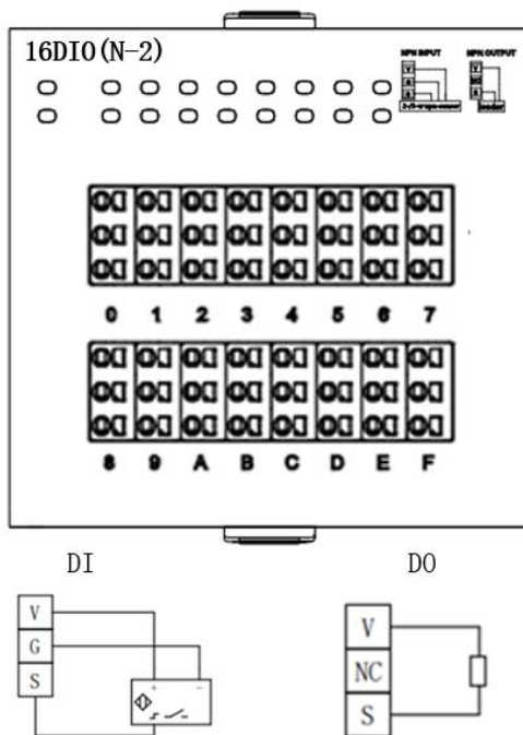
16DIO(N-2)
