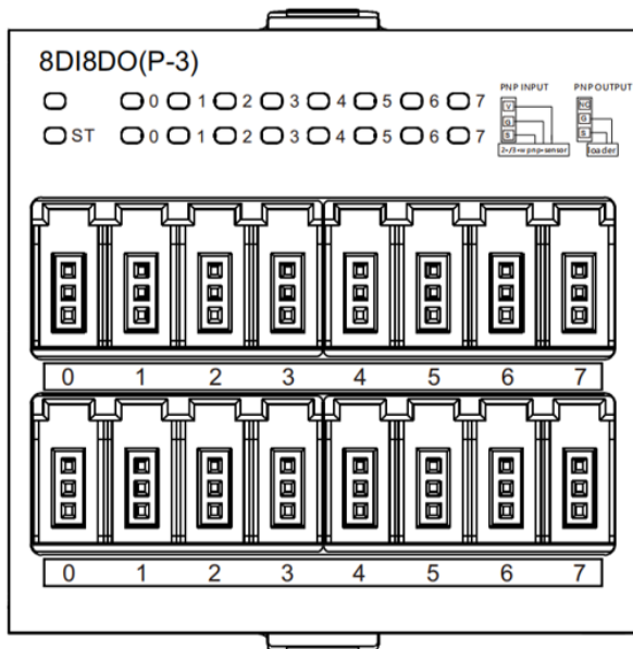
8DI8DO(P-3)
