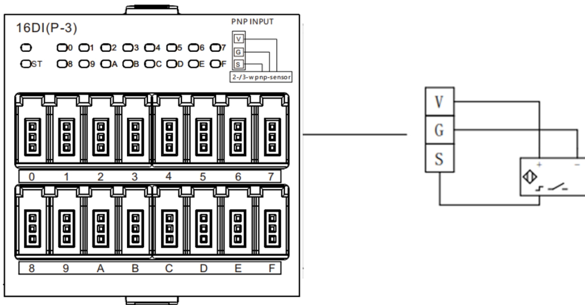
16DI(P-3)
