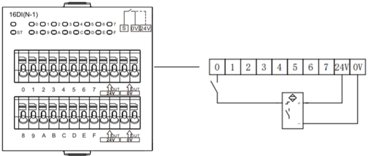
16DI(N-1)
